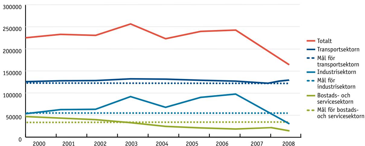
Koldioxidutsläpp från fossila bränslen CO 2 ton/år
