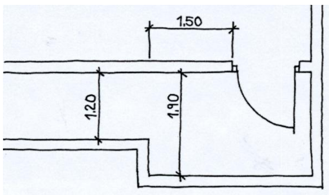
Bild 4. Exempel på dragvägs bredd vid riktningsändring.
