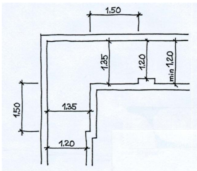
Bild 5. Exempel på dragvägs bredd vid riktningssändring.
