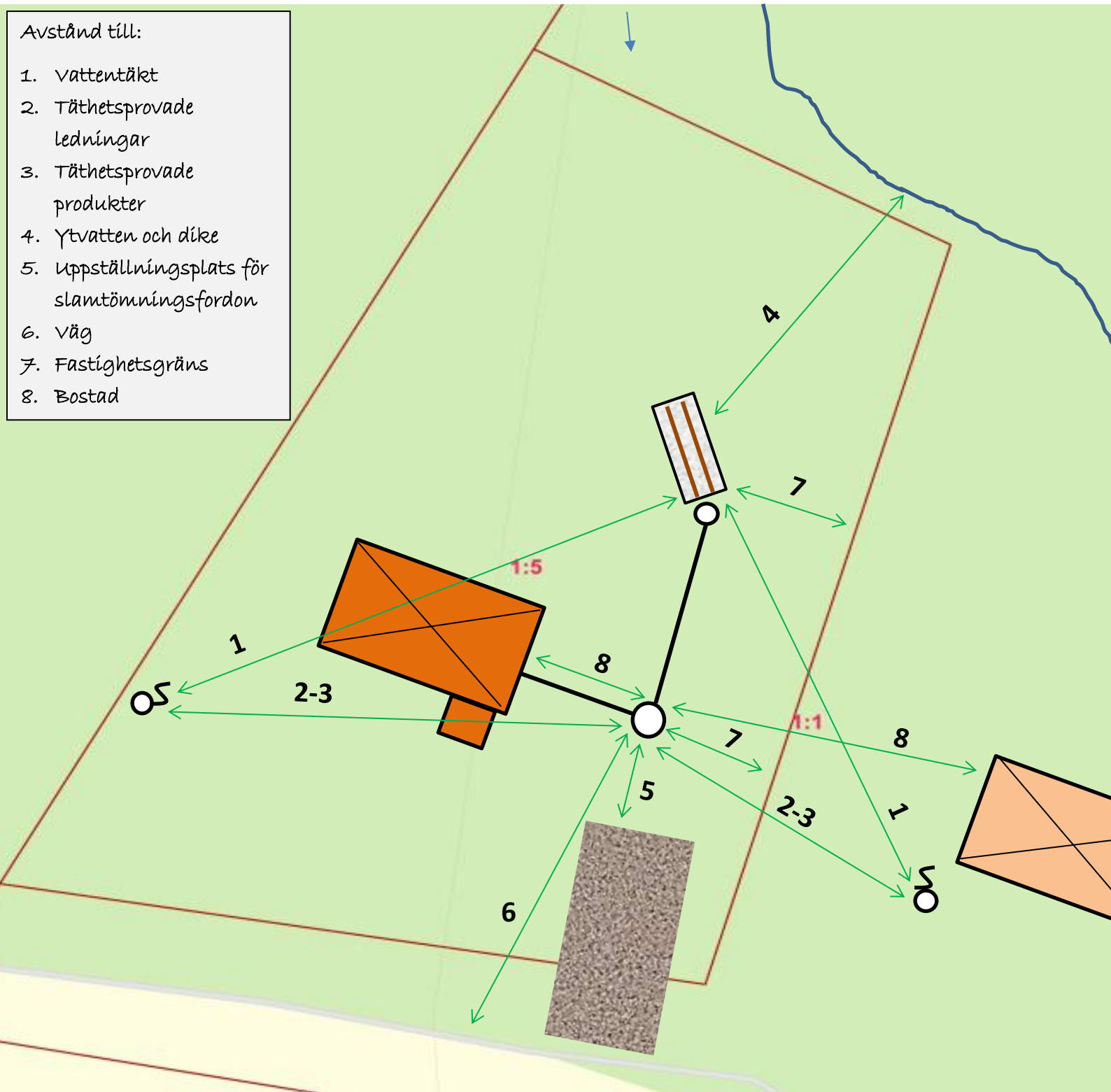
Figur 2. Horisontella skyddsavstånd
