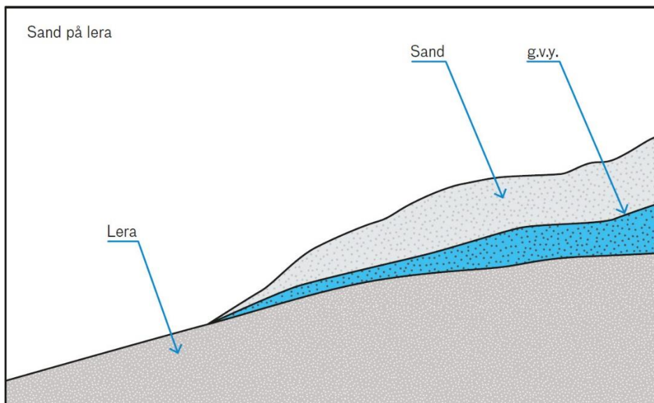
Figur 3. Planerar man att anlägga infiltrationen i ett jordlager med ett tätande lerlager (eller motsvarande) under, behöver mäktigheten på det jordlager som ska ta emot vattnet nedströms kontrolleras. G.v.y. är förkortning för grundvattenyta.
