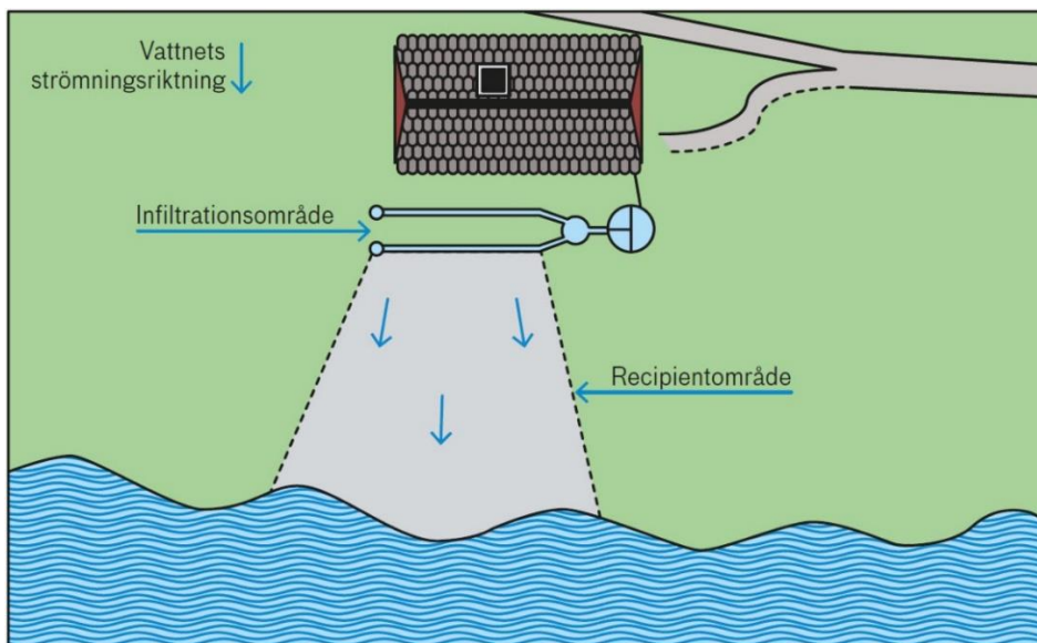
Figur 1. Recipientområdet nedströms anläggningen behöver ha förmåga att transportera bort det infiltrerade vattnet. Bilden är inte skalendig.
