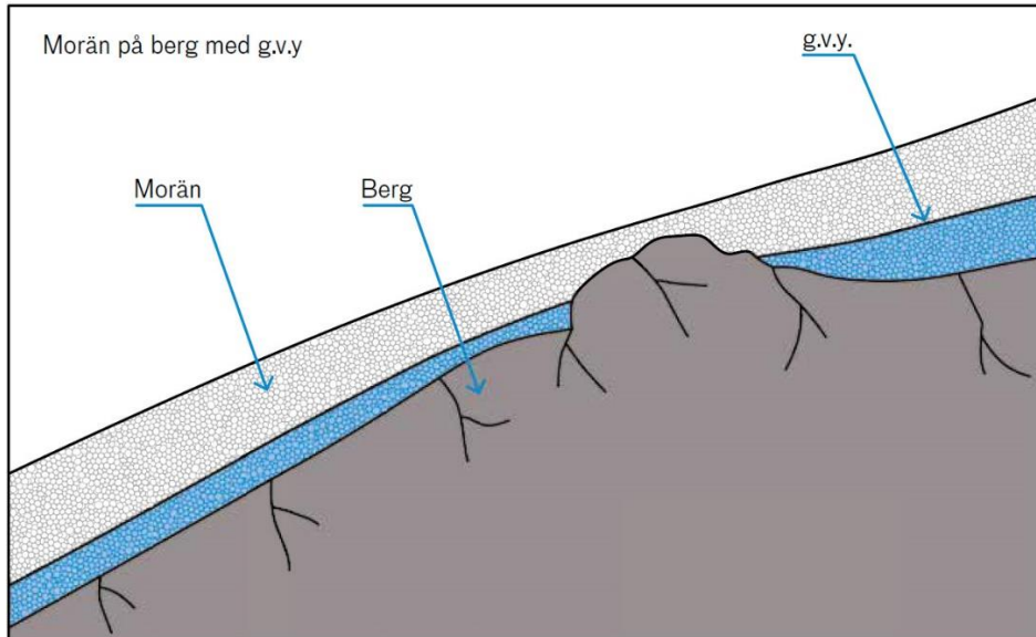
Figur 2. Om det är begränsat djup till berg finns anledning att undersöka utbredningen av olika jordlager. Då kan man behöva gräva flera provgropar. G.v.y. är förkortning för grundvattenyta.
