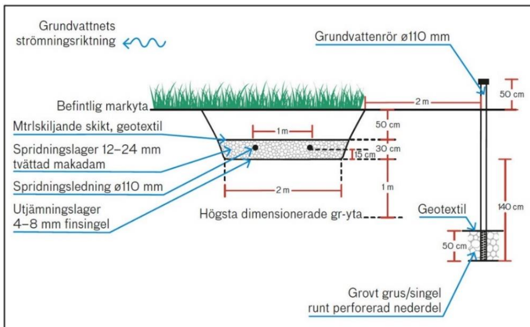
Figur 2. Exempel på tvärsnittsritning över infiltration med grundvattenrör för kontroll av grundvattennivå. Rörets botten bör ligga minst 140 cm under infiltrationsnivån (undre kanten på spridningslagret i detta exempel). Bifoga en tvärsnittsritning som underlag för installationsarbetet till din ansökan.
