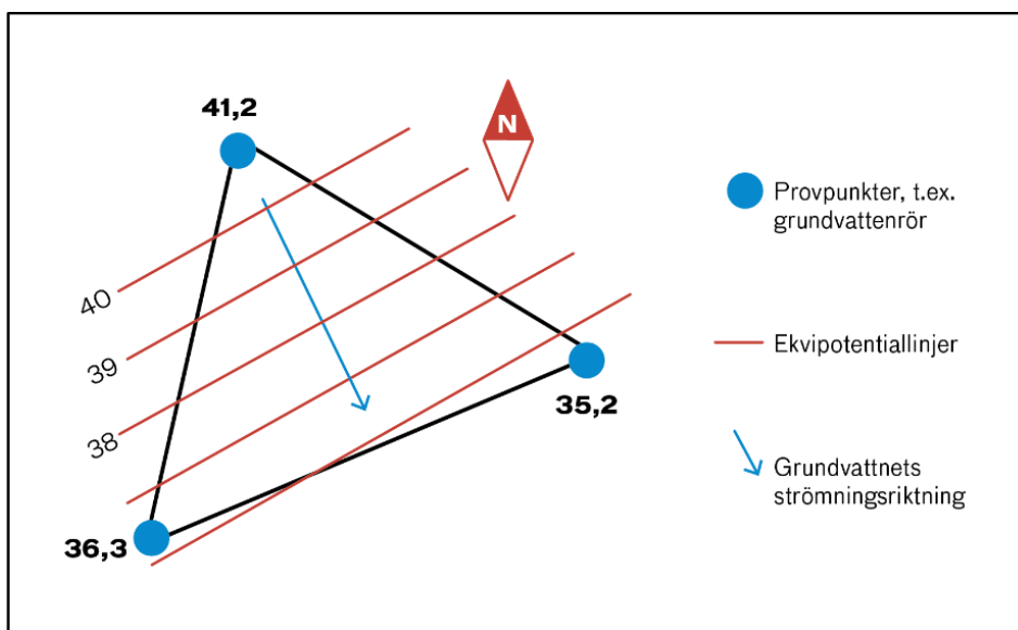
Figur 1. Grundvattnets strömningsriktning kan bestämmas med en så kallad "hydrologisk triangel" där nivåerna mäts i tre punkter. Strömningsriktningen (den blå pilen) ligger vinkelrätt mot ekvipotentiallinjerna (de röda linjerna).
