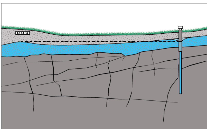
Figur 5. Bergborrad brunn i ett läge som balanserar mellan hög och låg risk. Brunnen ligger inte tydligt i avloppsvattnets strömningsriktning. Nivåskillnaden mellan brunnen och grundvattnet under avloppet är obetydlig. Bergets konduktivitet är acceptabel (större sprickighet och god tillrinning i brunnen). Det finns ett visst jorddjup och grundvattentillgången är tillräcklig för ett eller ett fåtal hushåll. En rimlig skyddsavståndsbedömning för detta fall kan vara 40–60 m.
