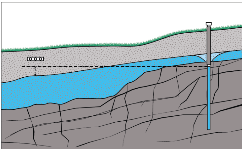
Figur 4. Bergborrad brunn med få riskfaktorer. Brunnen ligger tydligt högre i terrängen i förhållande till avloppet. Nivåskillnaden mellan brunnen och grundvattnet under avloppet är på rätt håll och betryggande. Bergets konduktivitet är hög (större sprickighet och god tillrinning i brunnen). Jorddjup och grundvattentillgång är betryggande. En rimlig skyddsavståndsbedömning för detta fall kan vara 30–40 m.
