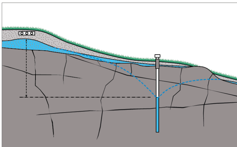
Figur 6. Bergborrad brunn med många riskfaktorer. Brunnen ligger i avloppsvattnets strömningsriktning, jorddjupet är dåligt, nivåskillnaderna mellan brunnen och grundvattnet under avloppet är stort och omvänt mot vad som är önskvärt. Bergets konduktivitet är låg (begränsad sprickighet och dålig tillrinning i brunnen) och grundvattentillgången i jordlagren är sparsam. En rimlig skyddsavståndsbedömning för detta fall kan vara 80–100 m.
