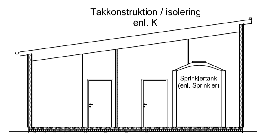
SEKTION A
